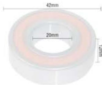
SV1465-B60042RS BALERO NTN TRASERO IMPULSOR NIPONDENSO 20mm ID x 42mm OD x 12mm W
