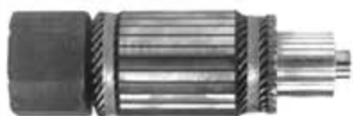
SV0155-A209124 ARMADURA BOSCH DEUTZ SCANIA 24V
